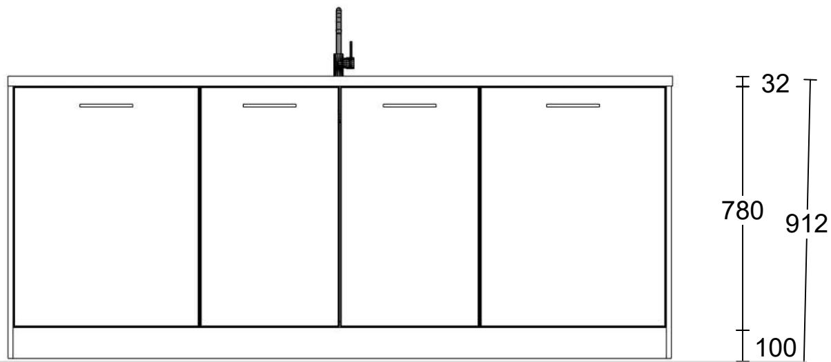
Vooraanzicht eiland
