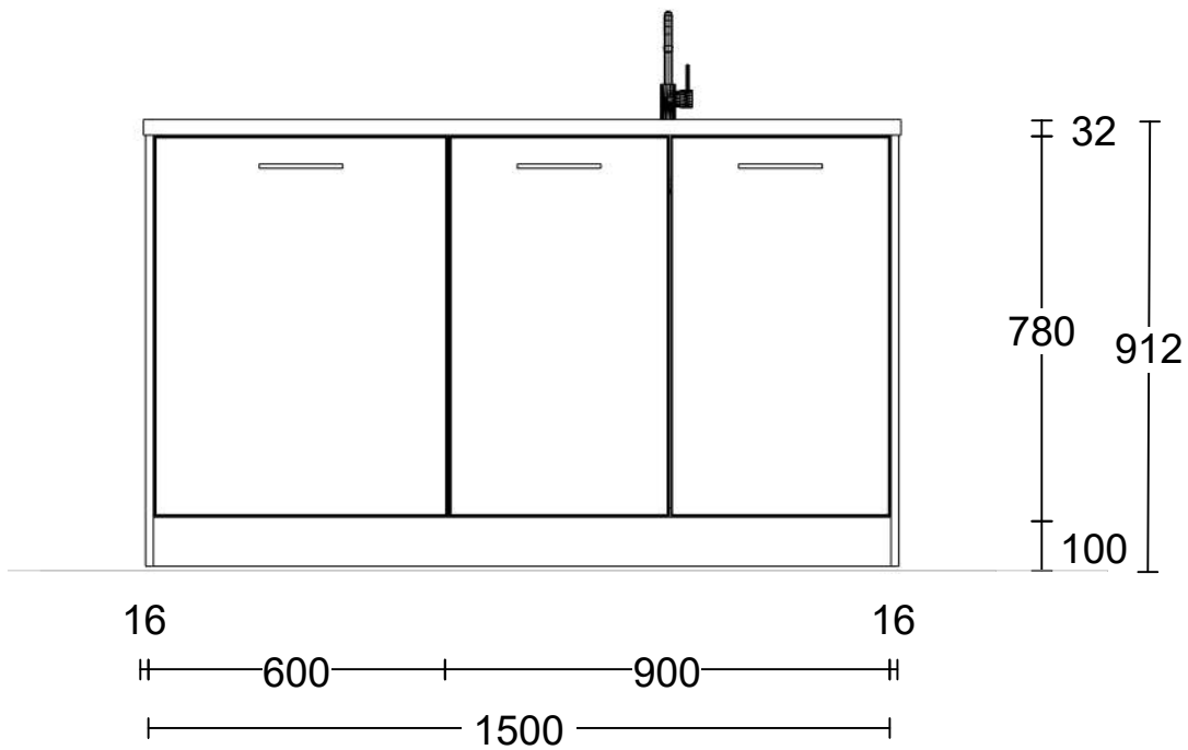
Vooraanzicht eiland
