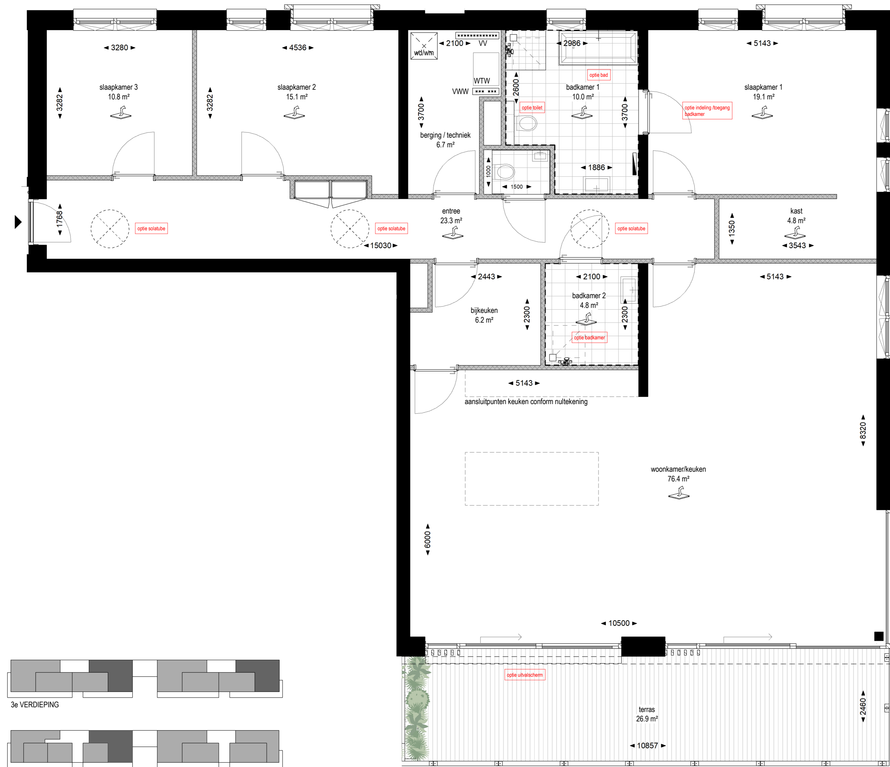
Optie type: Salix - M Plattegrond
